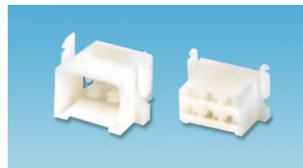
VF06 - 6 Way Connector
